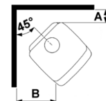
3440 installation d'angle
