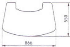
Contura 750, 750A Plaatstaal, dikte 1,5 mm Glas, dikte 6 mm
