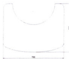
Contura 880 Plaat, dikte 1,5 mm Glas, dikte 6 mm
