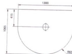
Contura 780/880 Draaihoek 90° Plaat, dikte 1,5 mm
