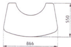
Contura 780 Plaatstaal, dikte 1,5 mm Glas, dikte 6 mm
